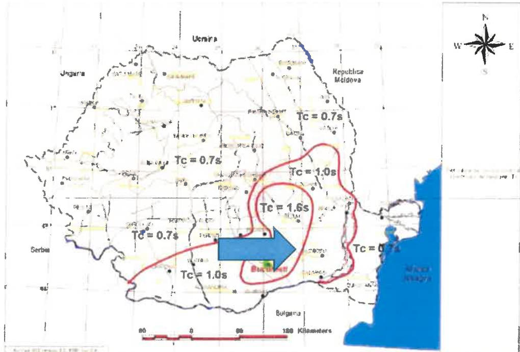
Fig.5 – Zona Teritoriului din punct de vedere al perioadei de control (colt) a spectrului de răspuns
