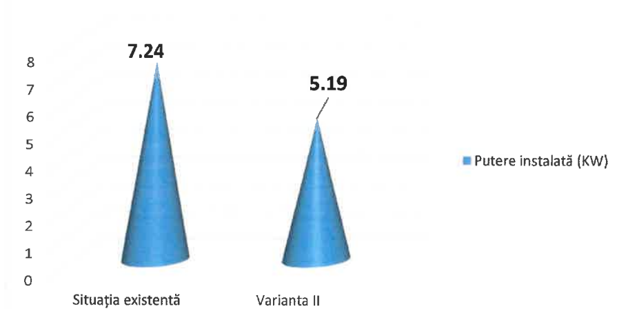
Fig. 14 Comparajie putere totală instalată
